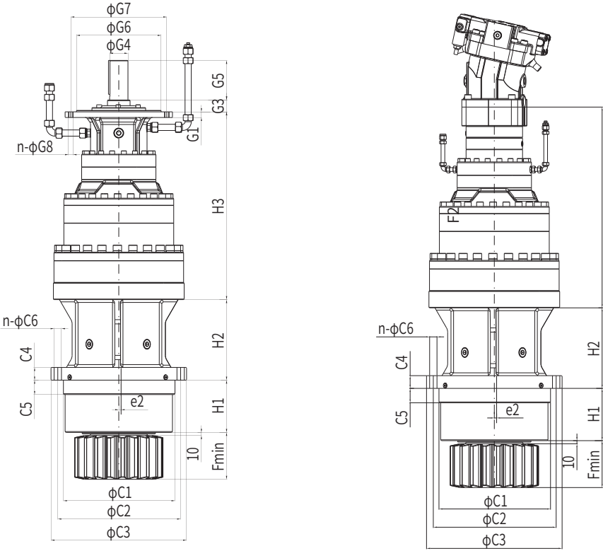
法兰B Flange B
