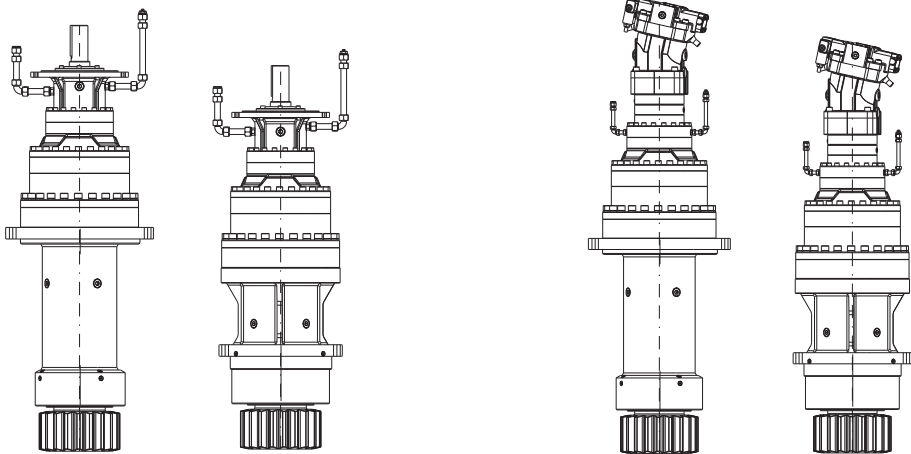
轴（电机）输入，竖直安装
