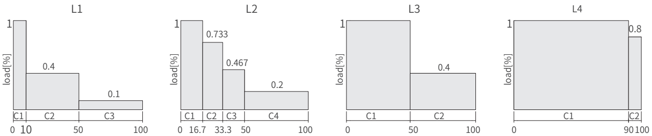
图3 起重机械典型载荷谱
