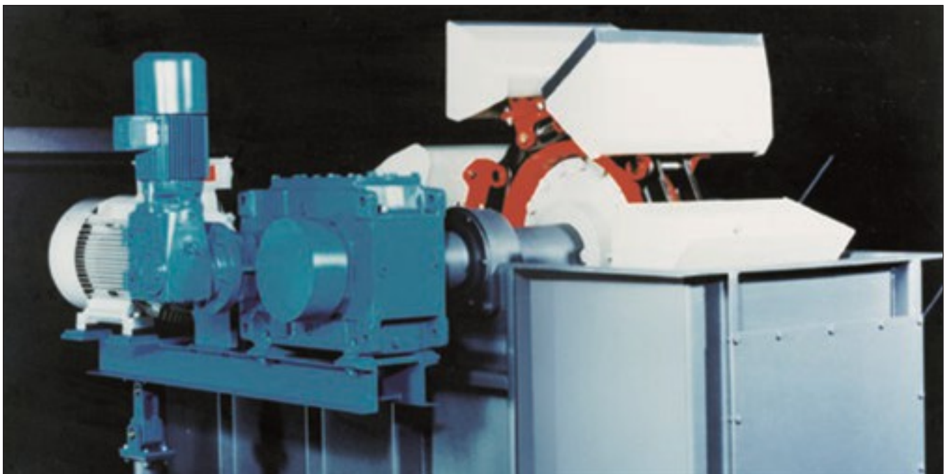
FLENDER-Zahnradgetriebe im Antrieb eines Becherwerks in der Zementindustrie
